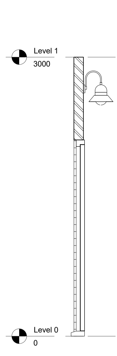
2 Section 1 1 : 20
